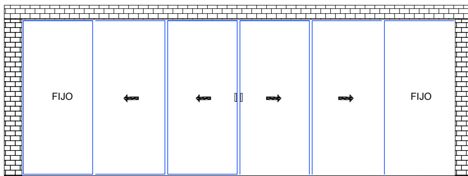
CABEZAL 2+1 = 1 FIJO 2 CORREDIZOS DOBLE
