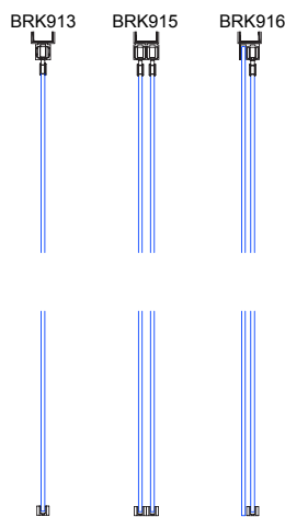
Corte transversal con rieles compatibles.
