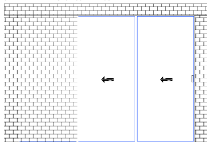
CABEZAL 2 + 1 = 1 MURO 2 CORREDIZOS
