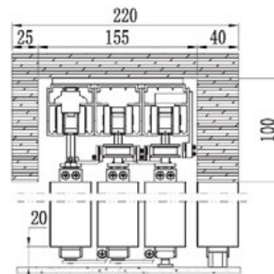
Vista transversal de la instalación general.
