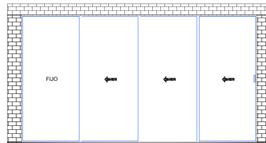
CABEZAL 3 + 1 = 1 FIJO 3 CORREDIZOS
